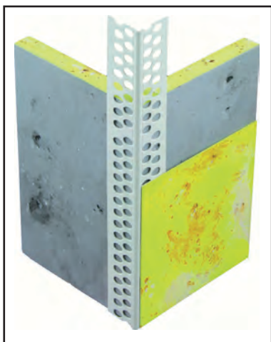
Eckprofil Genius PVC 24 x 24 mm
