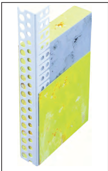
Rundbogenprofil Genius PVC 24 x 24 mm
