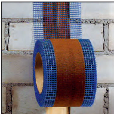
Stumpp-Armierungsgewebe Stuflex mit Isolierpapier
