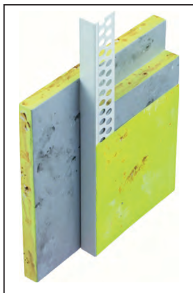
Lichtensteiner Profil Perfekt PVC 14 x 23 mm
