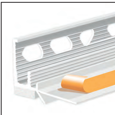
Anputzleiste mit elastischer Schutzlippe, einer zweiten Abzugskante und einem gelochten Einputzschenkel für zweilagige Putze T-FAL®
