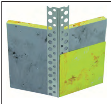
ALU-Kantenschutz für GK-Platten 135°
