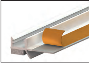
Anputzleiste mit elastischer Schutzlippe und flexiblem Abziehstreifen T-FAL®
